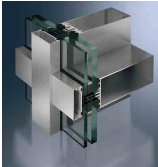
Schüco FW 80+ XR Schüco FW 80+ XR
